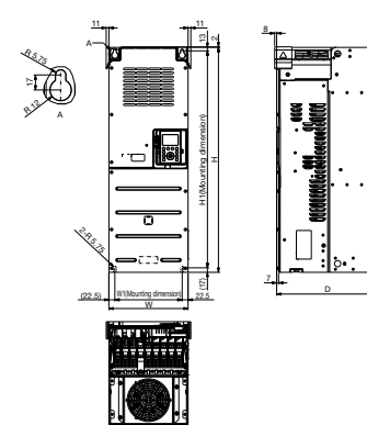
Frame Size A6
