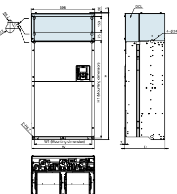
Frame Size A8
