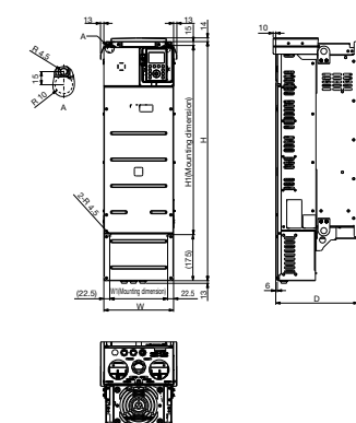
Frame Size A5
