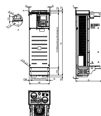
Frame Size A4
