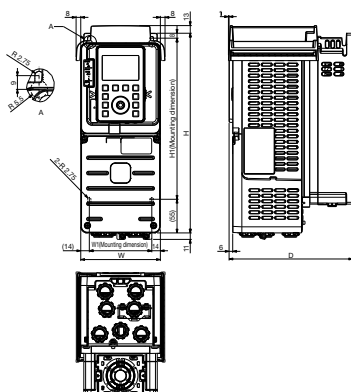
Frame Size A1
