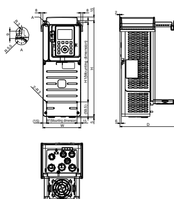
Frame Size A2
