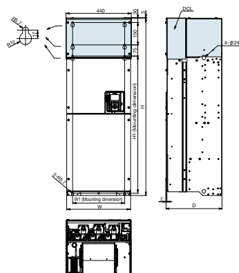
Frame Size A7
